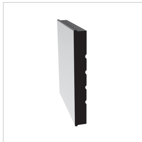
6-9/16" 9/16" X 6-9/16" 81-5/8"
